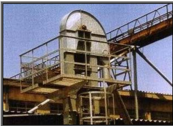
Elevátor ledobófej
