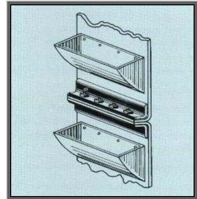
Végtelenítés fémpofillal
